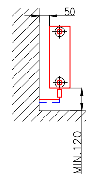
SCHÉMA UMÍSTĚNÍ TĚLESA
